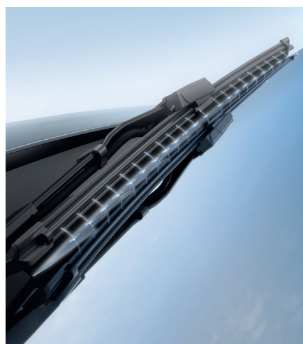
Das Aerotwin J·E·T Blade lenkt die Waschflüssigkeit punktgenau auf die Scheibe.
